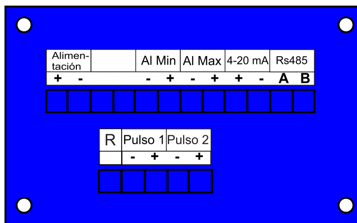
Definición de los símbolos de Cada Terminal
